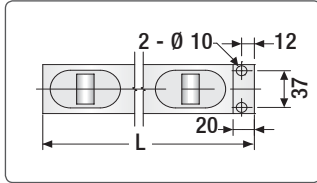
DL50 & DB50 Dış Ölçüleri
