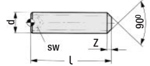
Inox Hex-socket Set Screw DIN 916 ISO 4029, A2-A4
