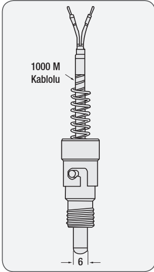
Bayonet Termokupl 6 - 8 mm'lik Rakorlu Sipariş Kodu: RT 2
