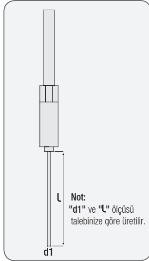
Mantel Termokupl Sensör Ucu: Ø4 mm Sipariş Kodu: MT 015
