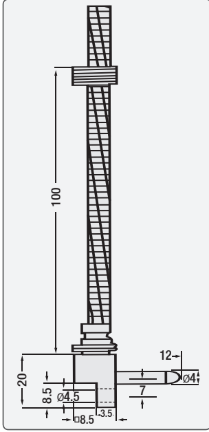
Açılı Termokupl Sensör Ucu: Ø4 mm Sipariş Kodu: TEWSH 17
