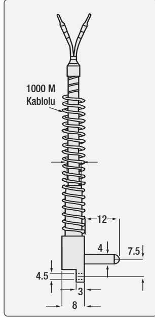
Açılı Termokupl Sensör Ucu: Ø4 mm Sipariş Kodu: RT 1
