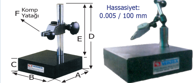
Gr.0 Hassasiyet
