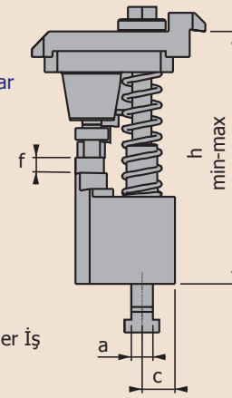
Ürün Nr.1270 Modüler (Desteksiz) Askı Pabuç
