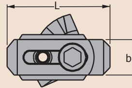
Ürün Nr.1230 Basamaklı Kombine Pabuç
