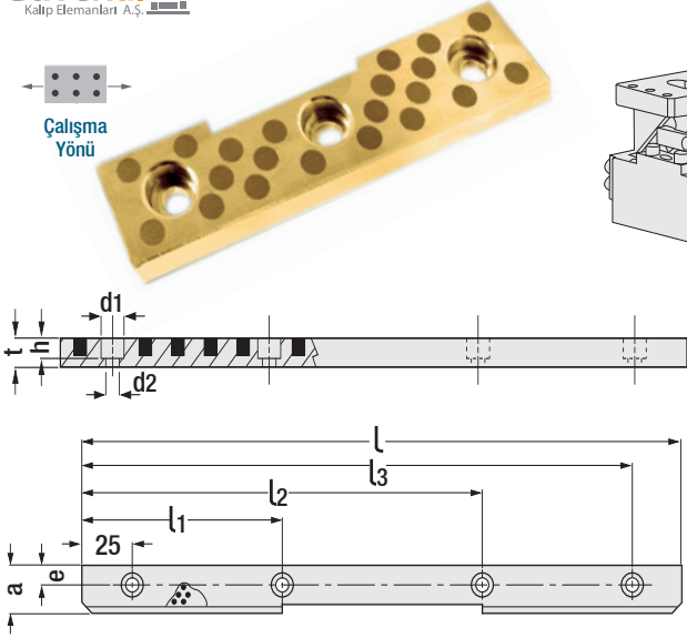
Kod: G 138 Grafitli, Değiştirilebilir Bronz Plaka
