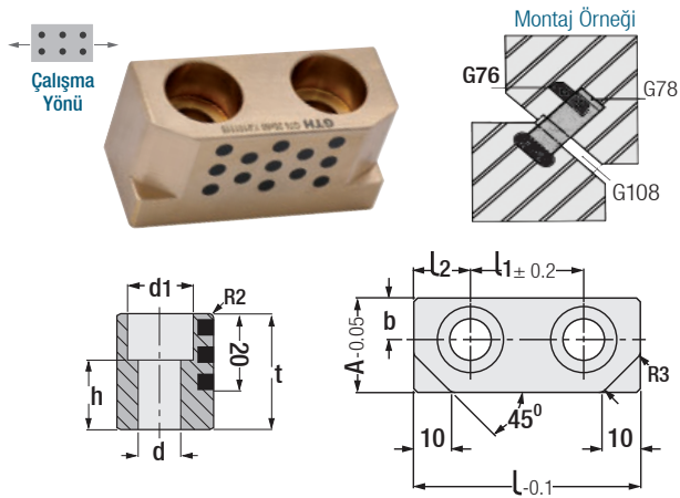
Kod: G 76 Grafitli, Sabit Dönüş Kam Plakası
