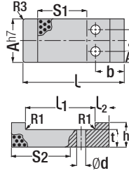
Grafitli, Bronz Kam Plaka
